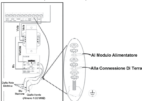
Figura 3-10: Schema di Cablaggio dell'Alimentatore
