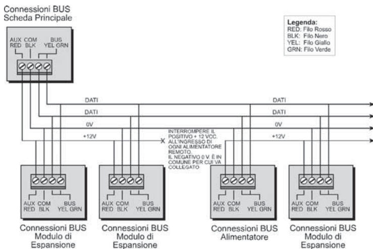
Figura 3-1: Morsettiera per le connessioni BUS
