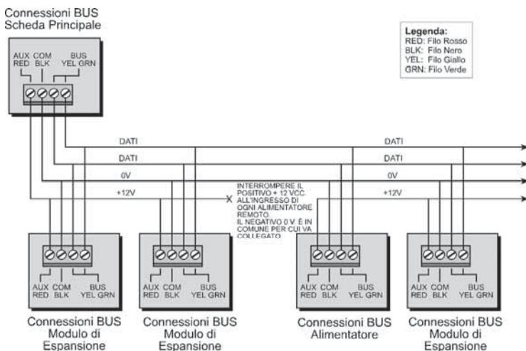
Figura 2-7: Morsettieria per le connessioni bus
