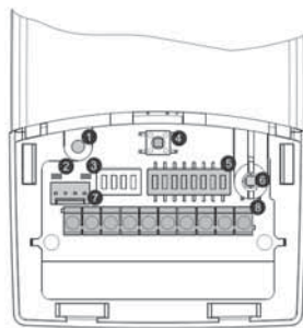
Schema del Ricevitore (senza coperchio)
