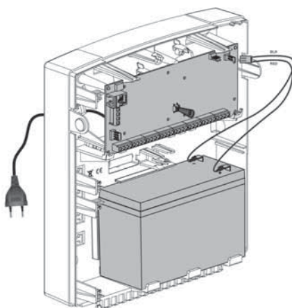
Figura 2-13 Posizionamento e collegamento della batteria
