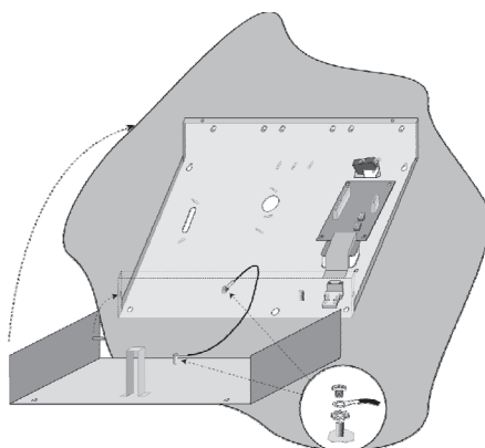
Figura 3-9: Modulo Alimentatore all'interno del Contenitore Metallico
