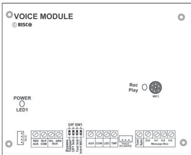
Figura 3-11: Scheda elettronica del Modulo Vocale
