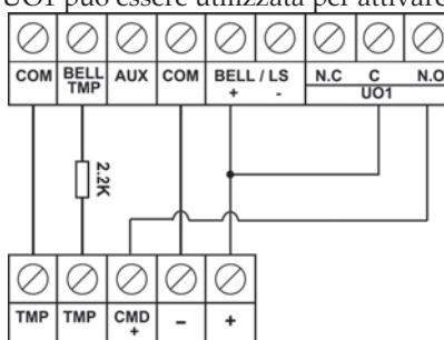
Figura 2-8: Cablaggio UO1 per una sirena autoalimentata
