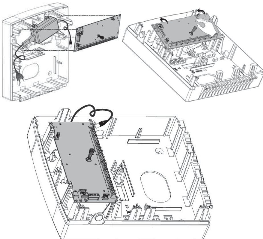
Figura 2-4 Posizionamento della scheda principale
