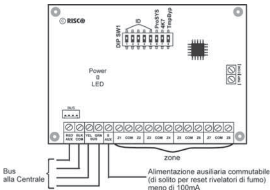
Figura 3-2: Espansioni zone scheda e schema di montaggio
