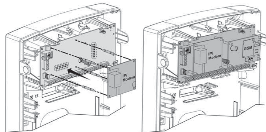
Figura 2-11 Posizionamento del modulo IP
