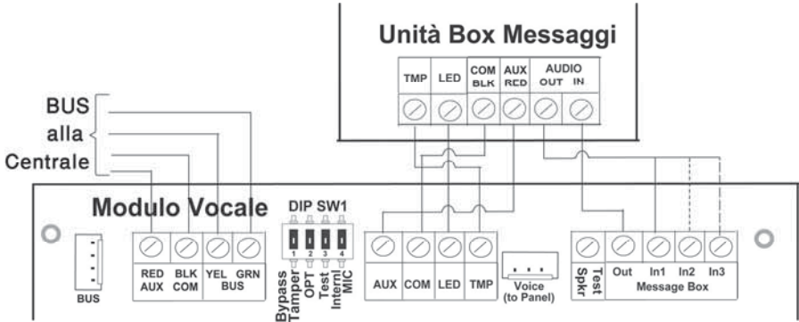
Figura 3-12: Cablaggio Modulo Vocale — Box Messaggi
