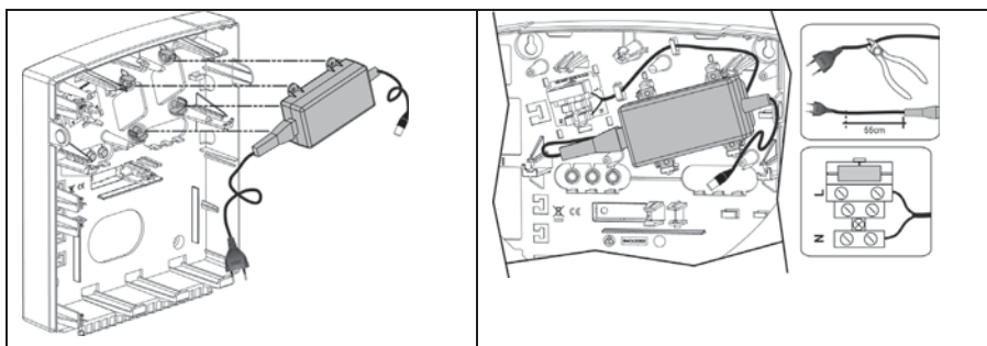
Figura 2-3 Posizionamento dell'alimentatore
