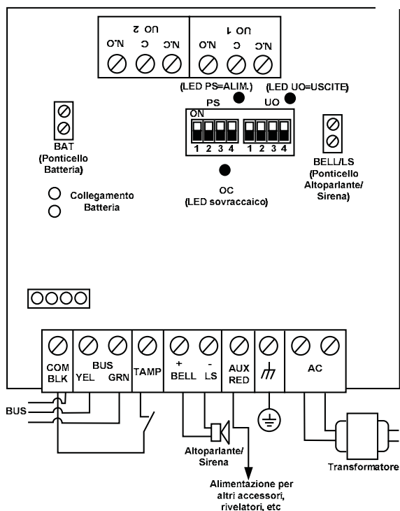
Figura 3-8: Vista Generale dell'Alimentatore Supplementare da 3Amp.
