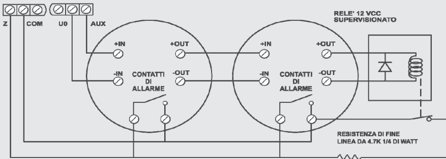
TIPICO CABLAGGIO DI UNA ZONA INCENDIO (DUE RILEVATORI DI FUMO A 4 FILI)
