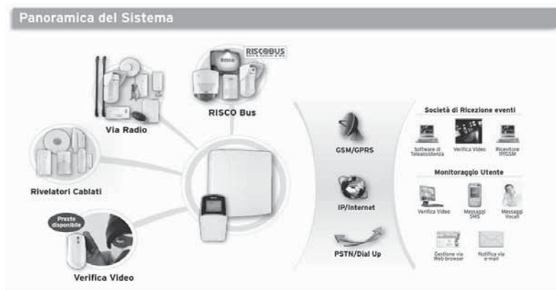
Figura 1-1 Architettura LightSYS
