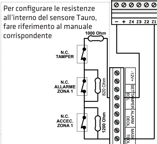
CONTATTO N.C. DI ALLARME ZONA 1, CONTATTO N.C. DI ACCECAMENTO ZONA 1 E CONTATTO N.C. DI TAMPER CON RESISTENZA DI TRIPLO BILANCIAMENTO ALL'INTERNO DEL SENSORE
