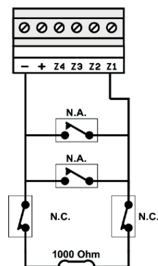
VARI CONTATTO N.A. E VARI CONTATTI N.C. CON RESISTENZA DI BILANCIAMENTO
