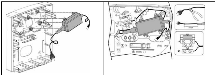
Figura 2-3 Posizionamento dell'alimentatore
