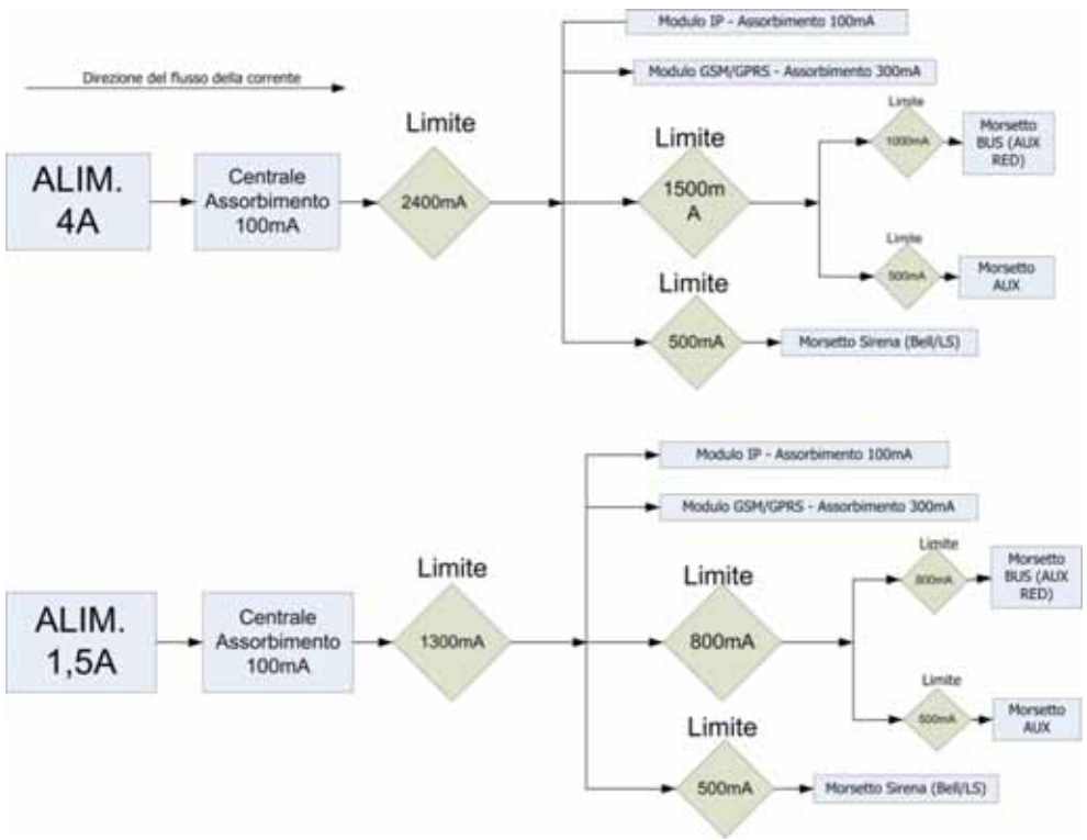
Connessioni BUS Scheda Principale
