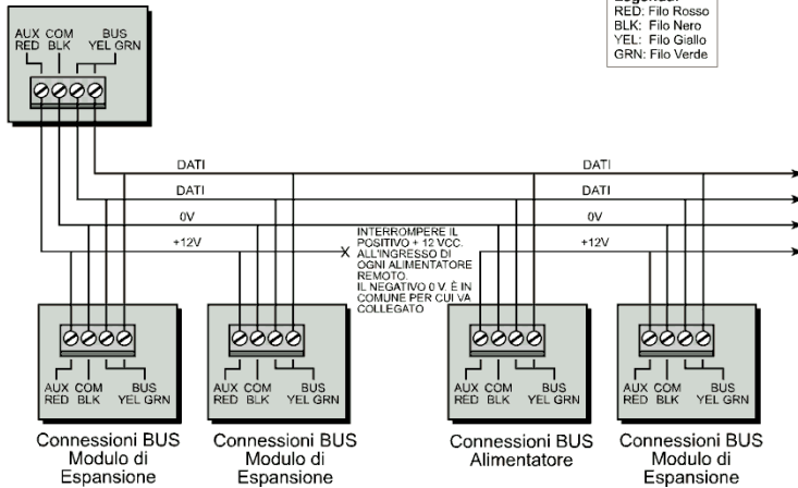
Figura 2-7: Morsettiera per le connessioni bus
