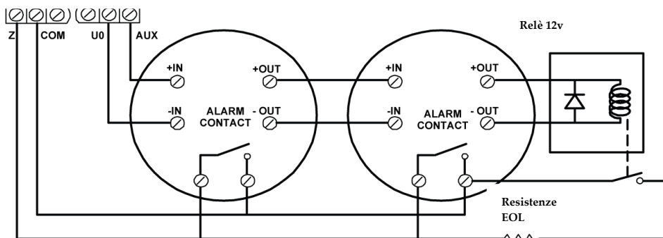
Cablaggio tipico rivelatori fumo 4 fili
